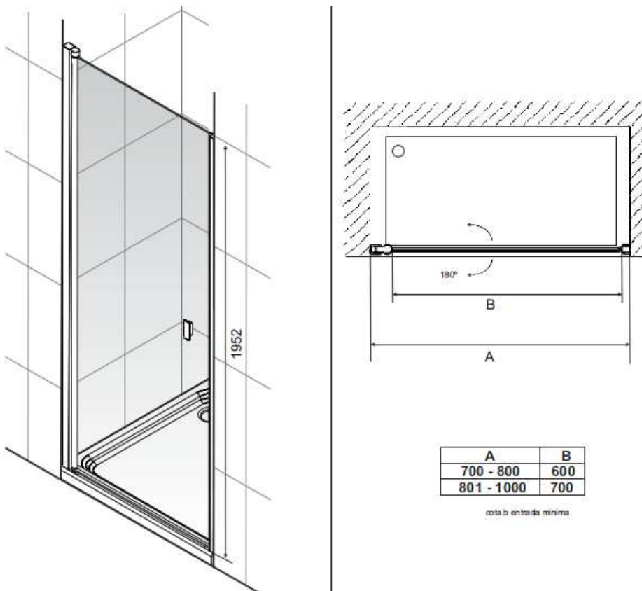
DBL1: FRONTAL DUCHA BATIENTE PARA LATERAL 1 HOJA
