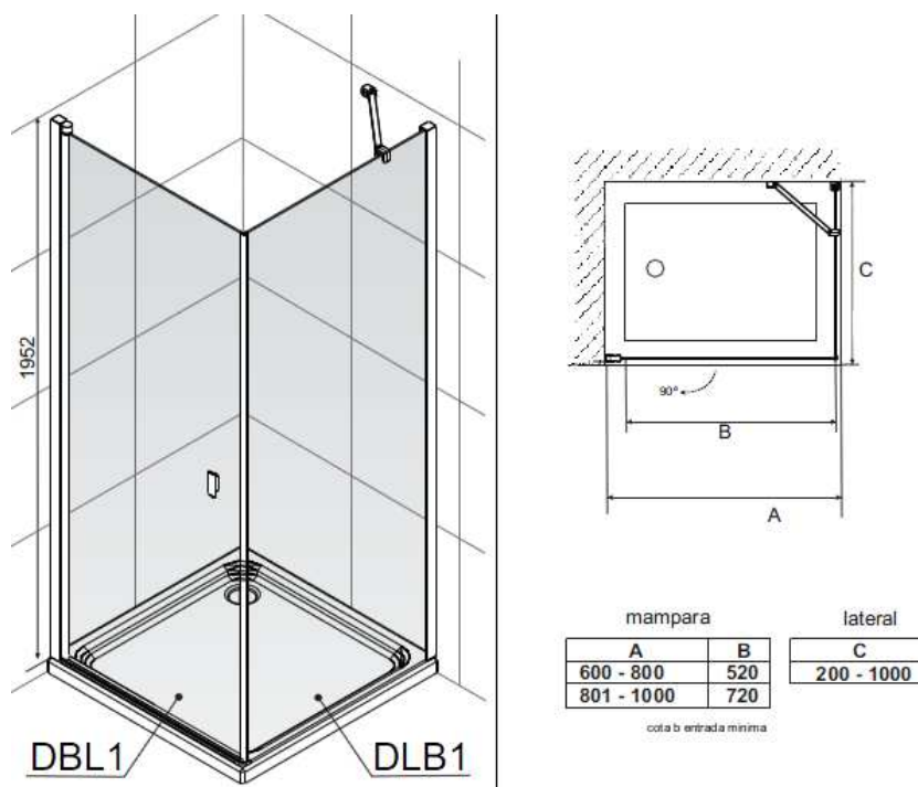
DBL1: FRONTAL DUCHA BATIENTE PARA LATERAL 1 HOJA
