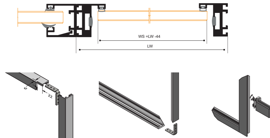
DETALLE DE UNIÓN DE MARCO 90°
