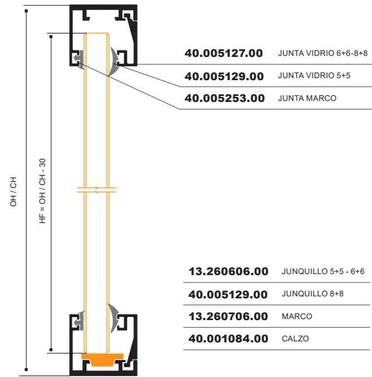
SECCIÓN A-A
